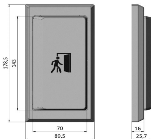
Рис. 1. Габаритные размеры
